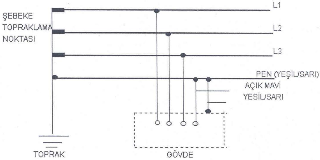
ŞEKİL 1-1 TÛMÜNDE KORUMA VE NÖTR İŞLEVLERİNİN YÛKLENDİĞİ TEK İLETKEN ÇEKİLMİŞ TN SİSTEMİ (TN-C)
