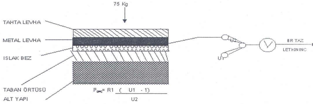
Şekil 20 – Zemin yalıtımlık direncinin ölçülmesi
